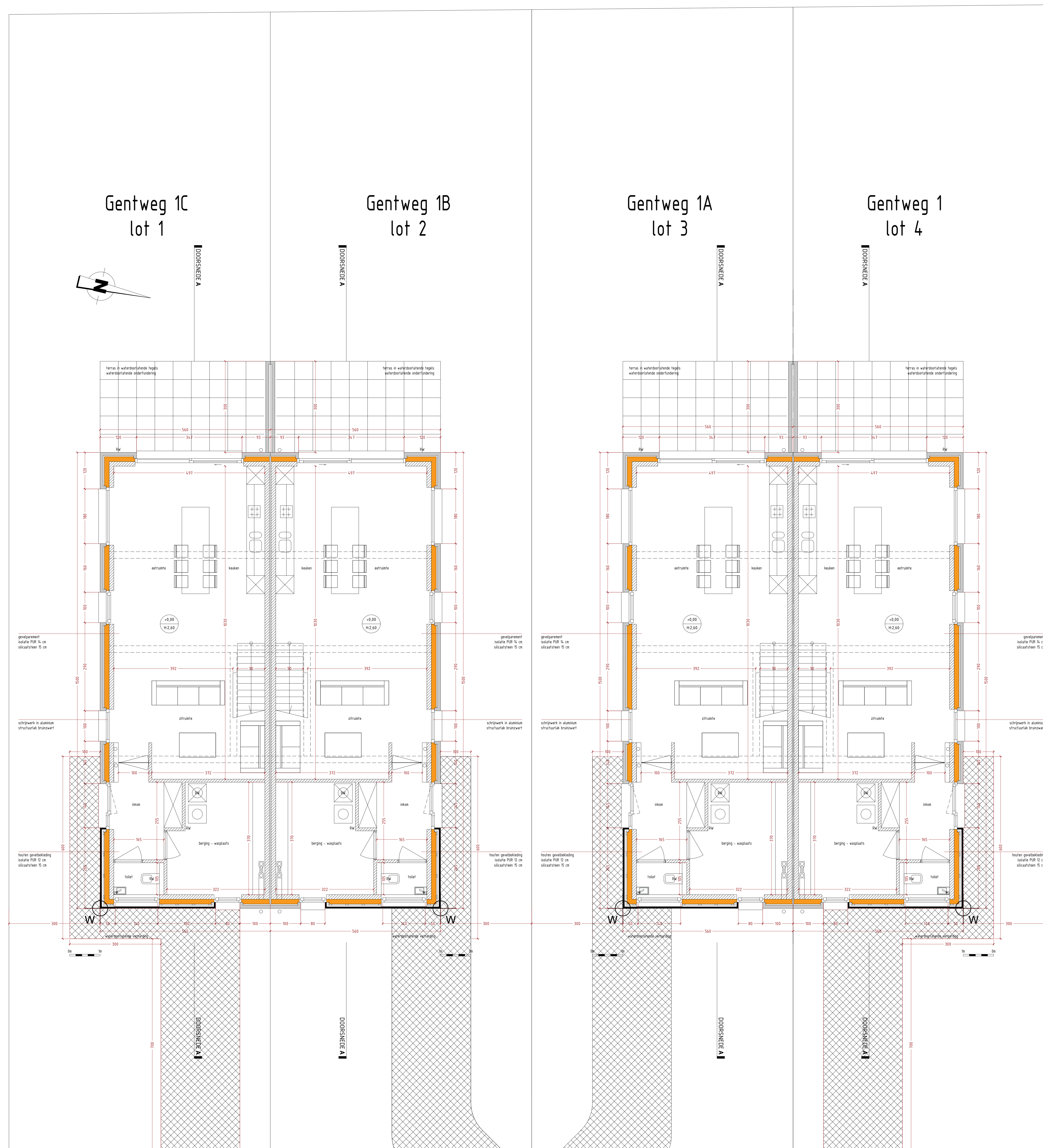
Plan gelijkvloers Nieuwe toestand
