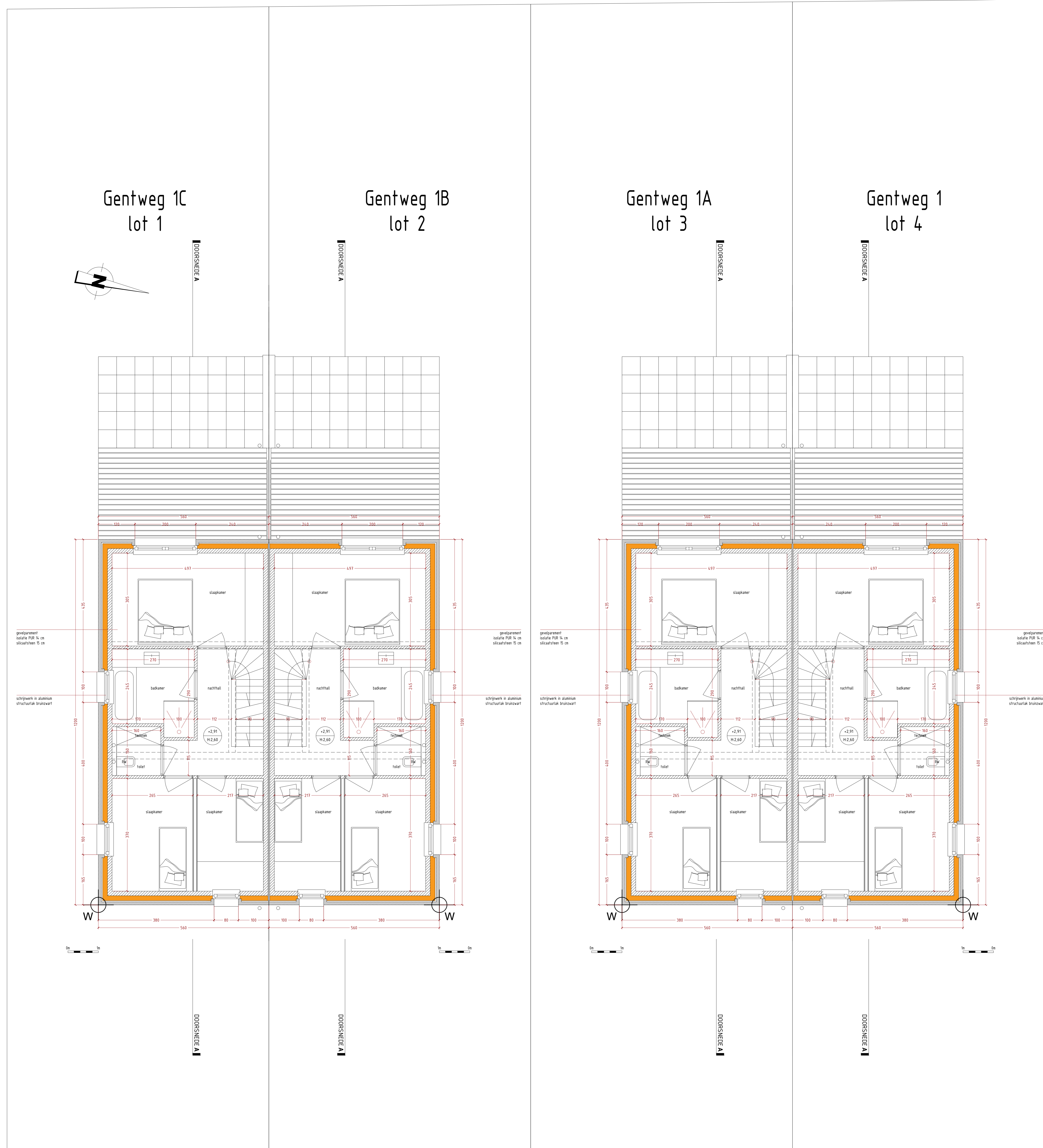
Plan verdieping Nieuwe toestand
